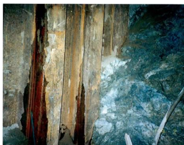
軟岩 鋼矢板貫入状況
